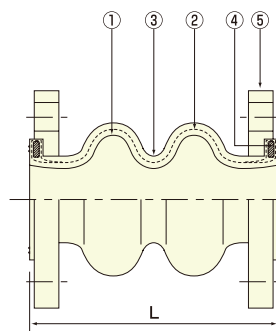
部品表 Parts List
