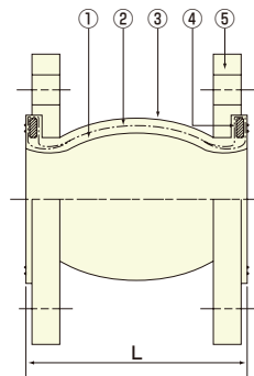
部品表 Parts List
