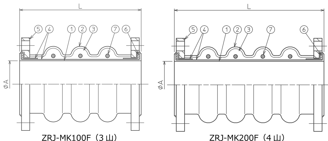
図1. 構造
