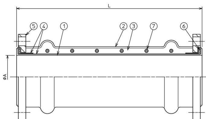
図1. 構造
